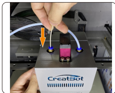
插入耗材
