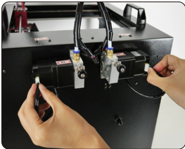
Plugin cable 1
